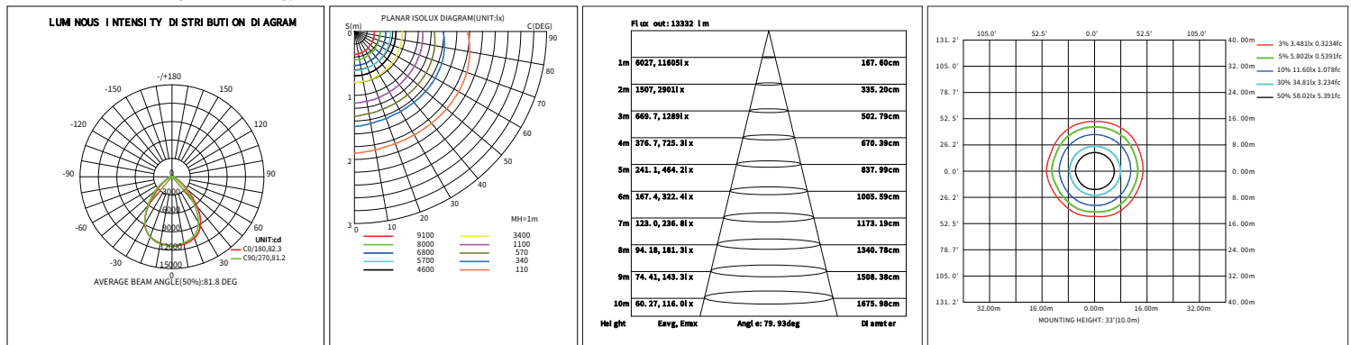
SS-UFO12-200W-H-TCP-[A,B,C,D,blank](200W-5000K)
