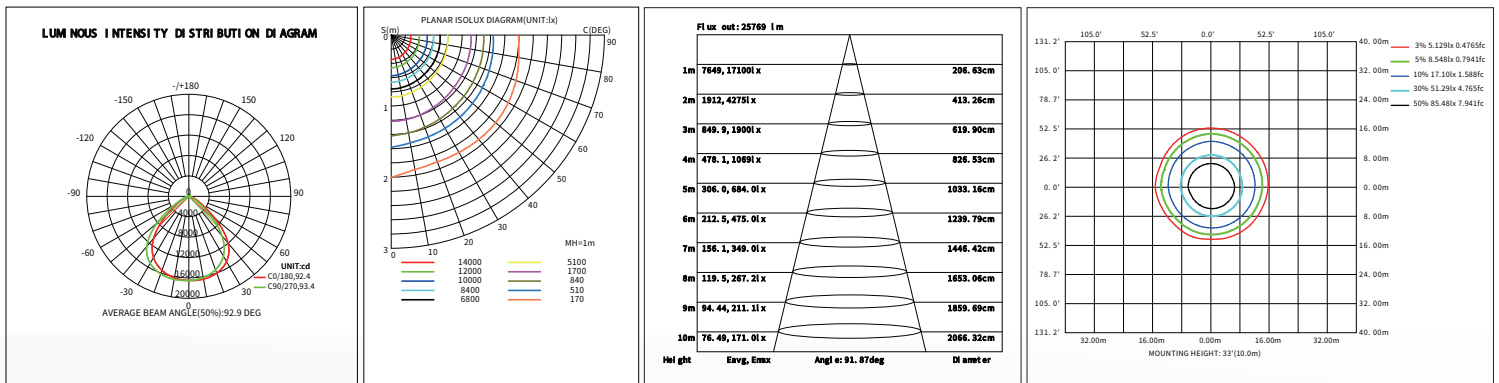
SS-UFO12-240W-H-TCP-[A,B,C,D,blank](240W-5000K)
